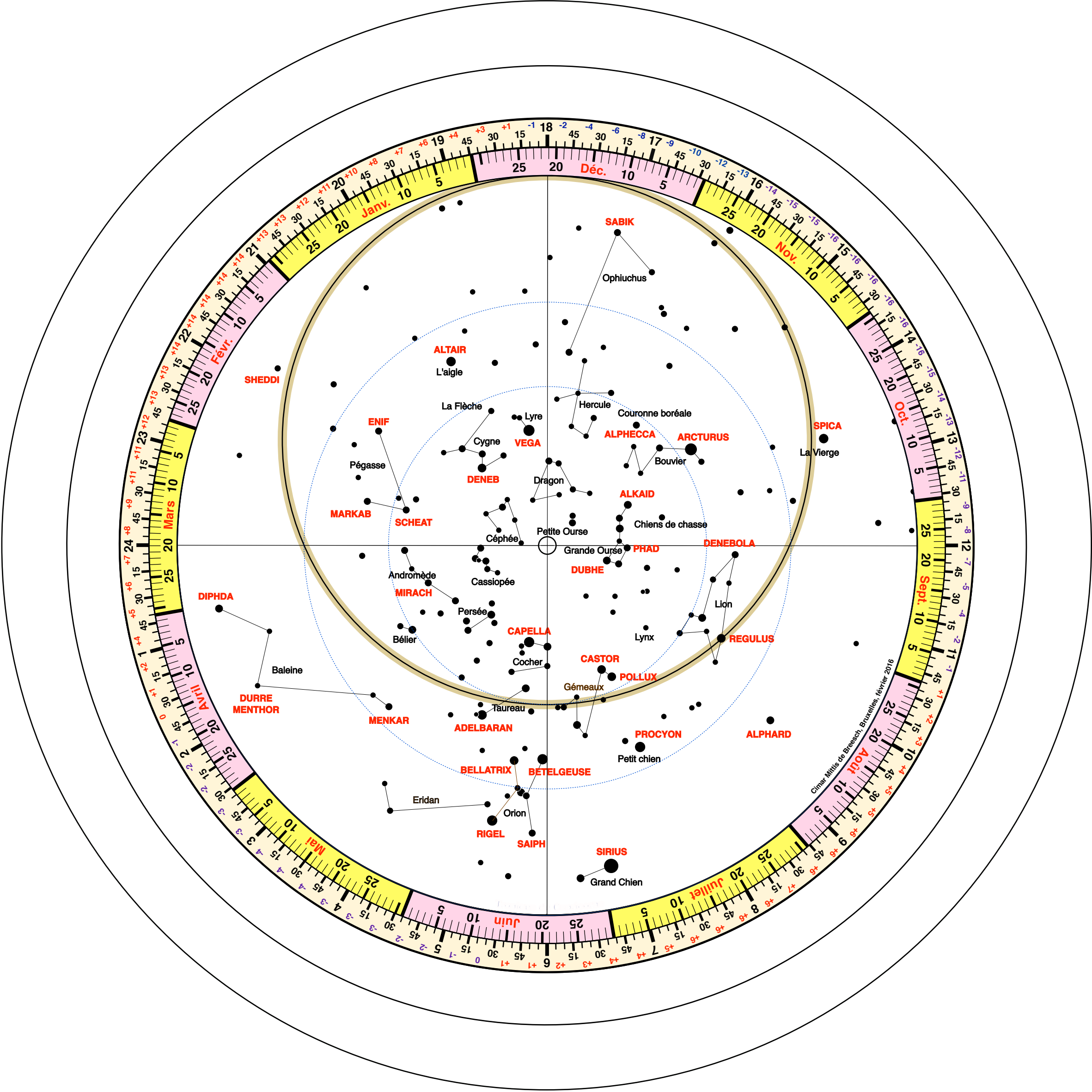
Découpe suivant cercle extérieur = astrolabe avec couronne heures moyennes Découpe suivant cercle intérieur = astrolabe sans couronne heures moyennes
